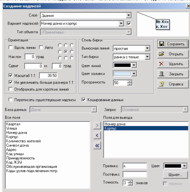
Рисунок 17.8. Создание варианта надписи “Номер дома и корпус”
