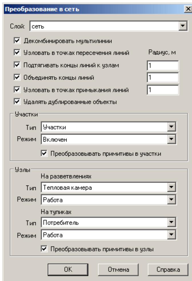
Рисунок 9.9. Диалог преобразования в сеть
