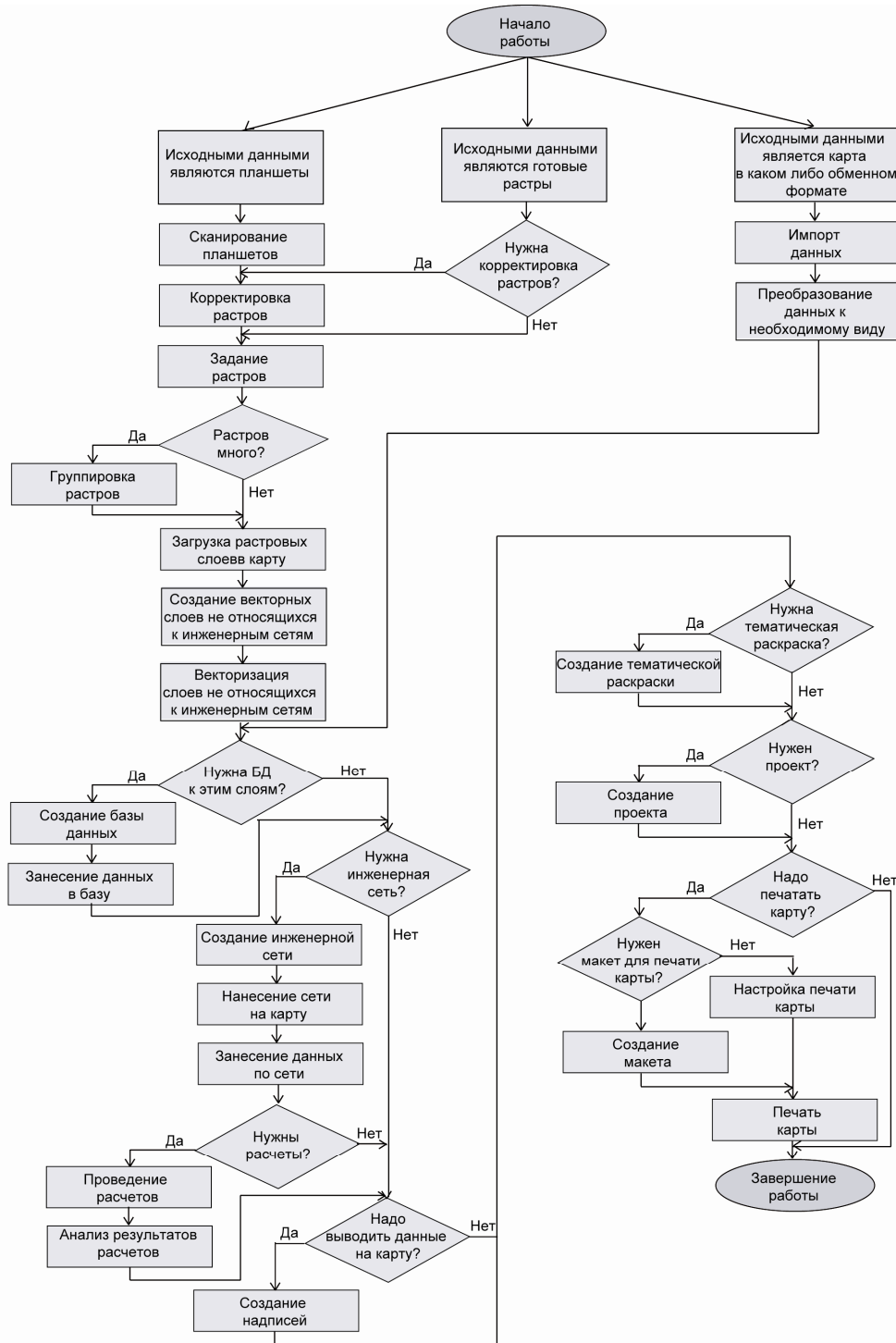
Рисунок 25.1. Алгоритм работы с системой
