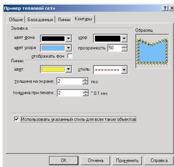
Рисунок 10.3. Окно настройки слоя. Вкладка Контур
