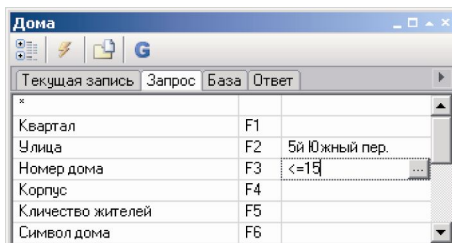
Рисунок 14.87. Пример создания запроса
