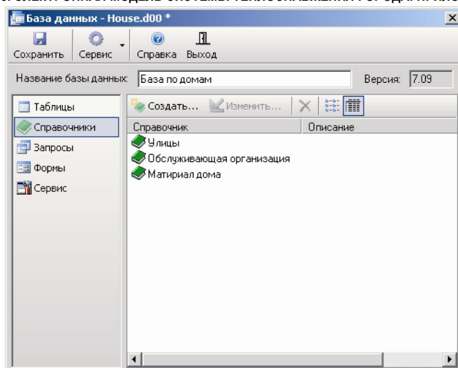
Рисунок 14.12. Окно редактора БД. Тип объектов – Справочники
