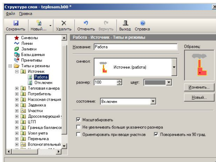
Рисунок 7.12. Вкладка с параметрами режима типового объекта
