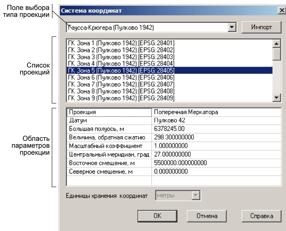
Рисунок 6.5. Диалог параметров проекции слоя
