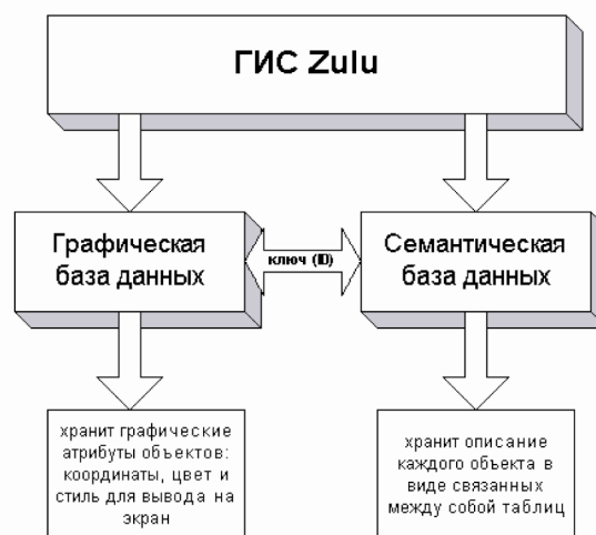
Рисунок 4.1. Структурная схема представления информации в системе Zulu
