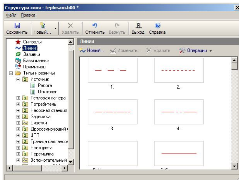
Рисунок 7.14. Раздел «Линии» диалога структуры слоя
