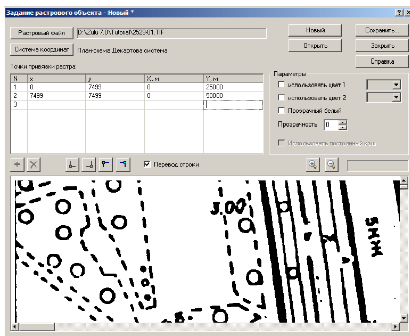
Рисунок 6.19. Задание растра
