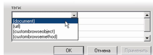
Рисунок 14.61. Установка Тэга
