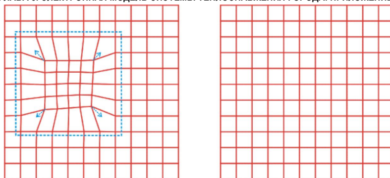
Рисунок 10.12.
