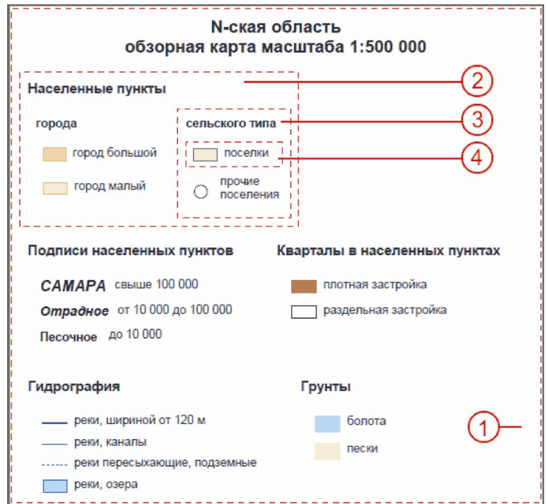
Рисунок 20.5. Структура легенды
