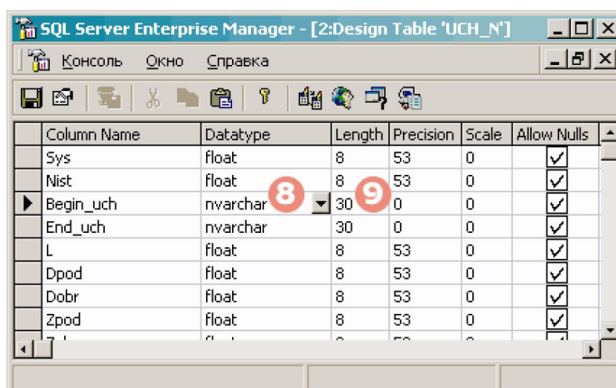
Рисунок 14.36. Структура таблицы
