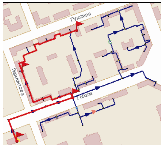
Рисунок 22.4. Нахождения пути
