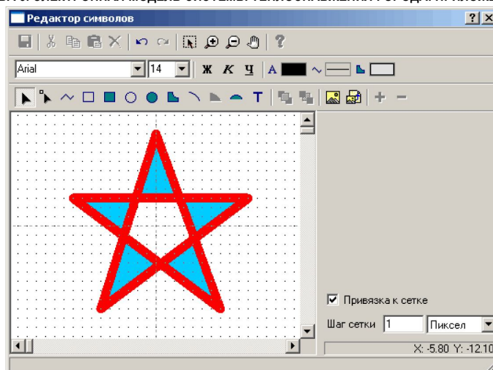
Рисунок 7.38. Редактор символов
