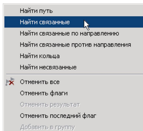
Рисунок 9.10. Контекстное меню
