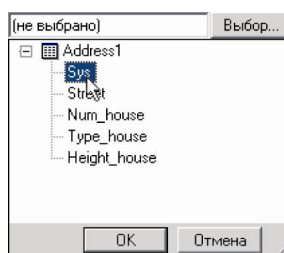
Рисунок 14.46. Выбор поля
