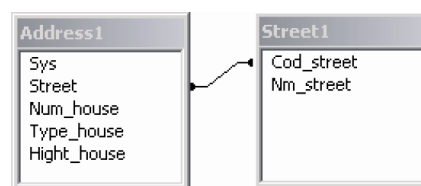
Рисунок 14.20. Связанные таблицы
