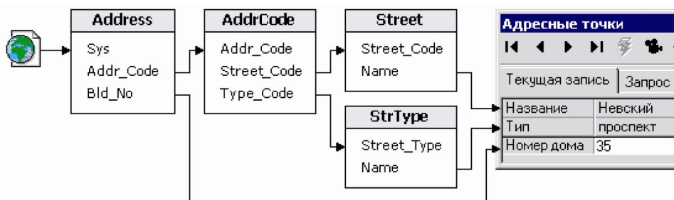
Рисунок 14.1. Схема данных
