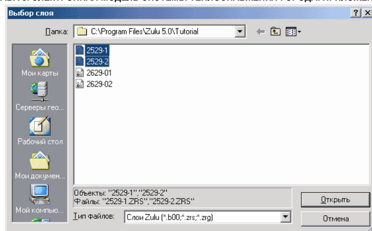
Рисунок 6.20. Выбор растра
