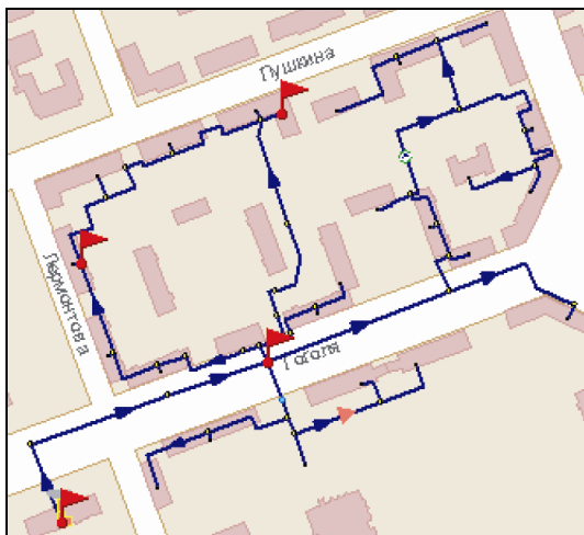
Рисунок 22.3. Нахождения пути
