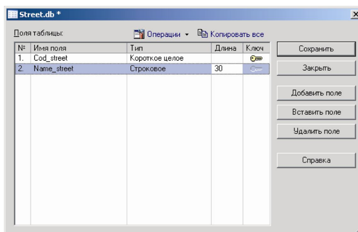
Рисунок 14.50. Создание таблицы
