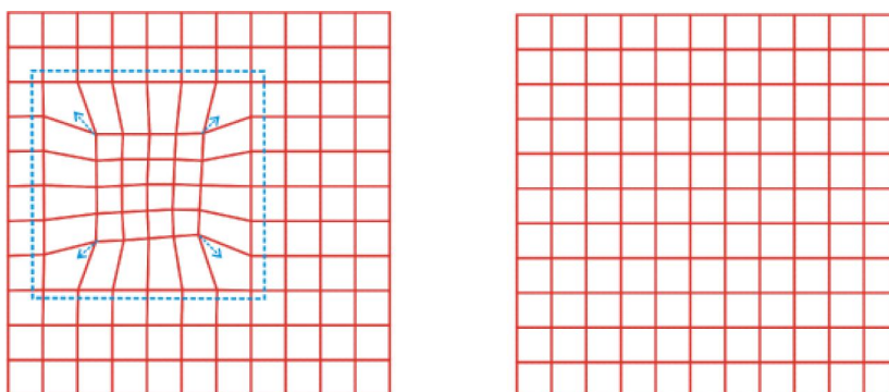
Рисунок 6.15.
