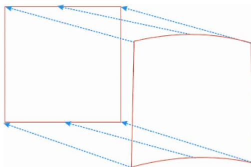
Рисунок 10.11.
