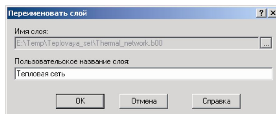
Рисунок 10.5. Диалоговое окно
