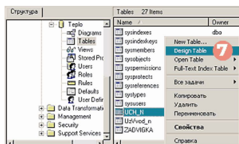
Рисунок 14.35. Контекстное меню
