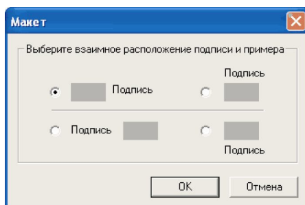
Рисунок 20.9. Диалог «Макет»
