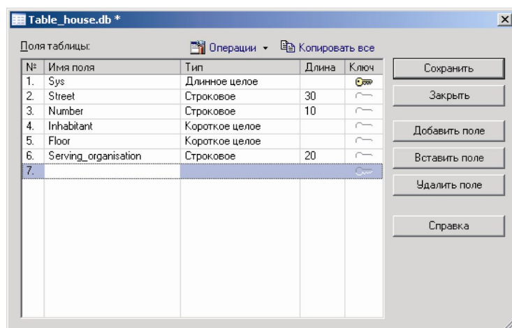
Рисунок 14.4. Диалоговое окно создания таблицы
