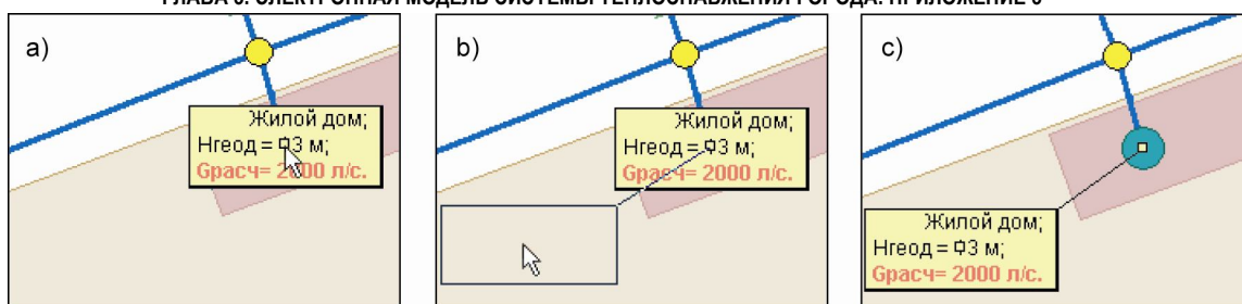
Рисунок 17.5. Перемещение надписи
