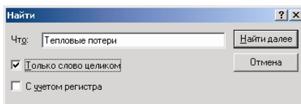
Рисунок 5.3. Панель поиска
