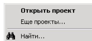
Рисунок 5.6. Контекстное меню
