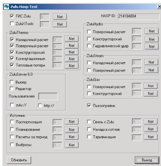
Рисунок 28.6. Конфигурация ключа
