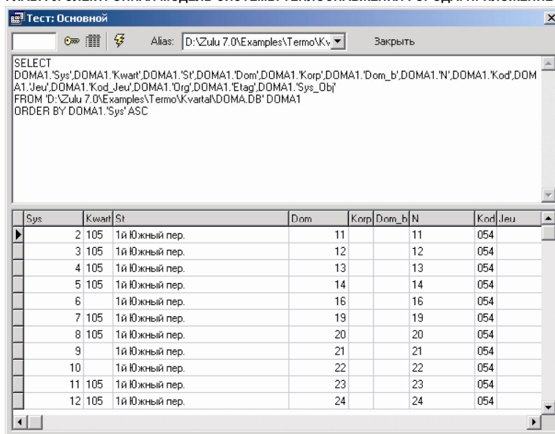
Рисунок 14.22. Окно Запрос
