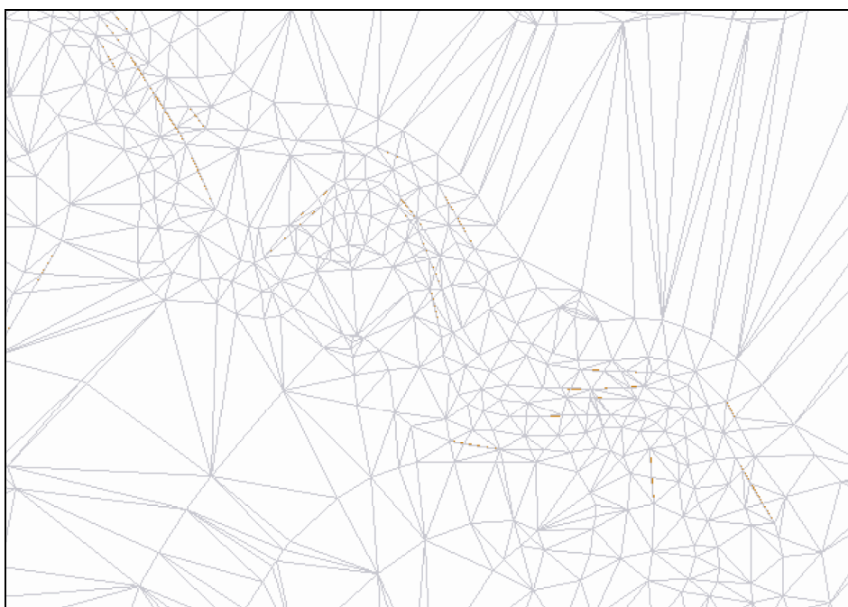
Рисунок 13.3. Модель рельефа
