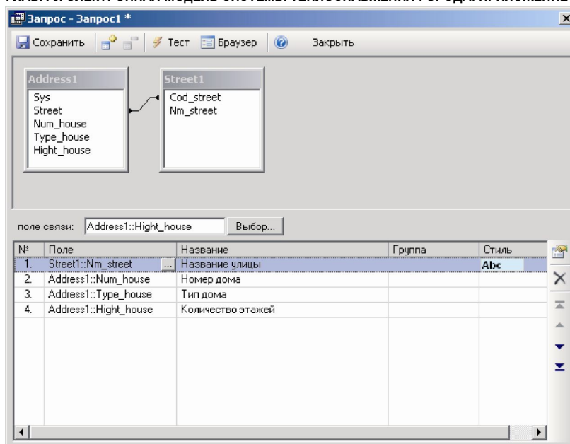
Рисунок 14.51 Создание запроса
