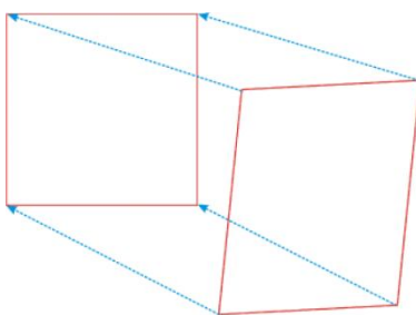
Рисунок 6.13.
