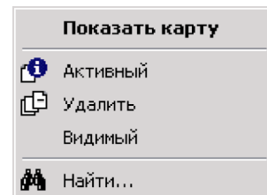
Рисунок 5.8. Контекстное меню
