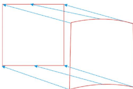
Рисунок 6.14.
