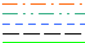
Рисунок 7.15. Векторная штриховка
