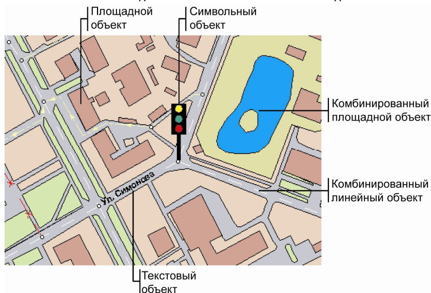
Рисунок 4.5. Примеры объектов
