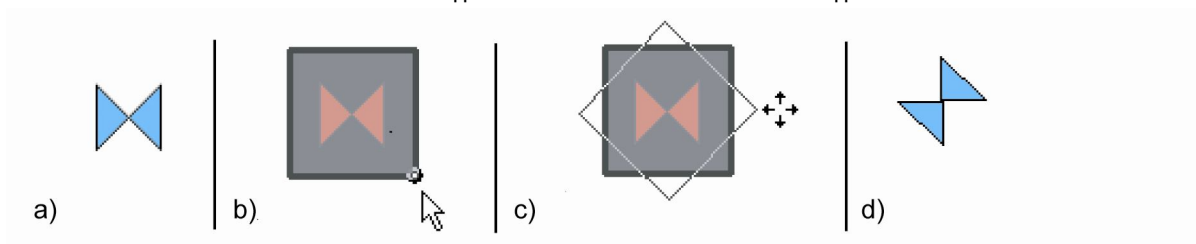
Рисунок 8.20. Поворот символа
