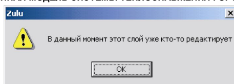
Рисунок 10.14. Окно предупреждения
