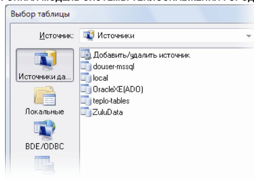
Рисунок 14.11.
