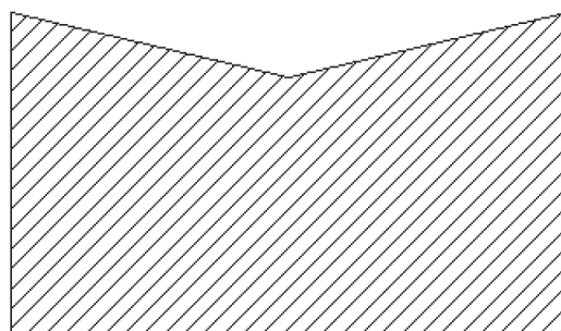
Рисунок 7.29. Векторная штриховка
