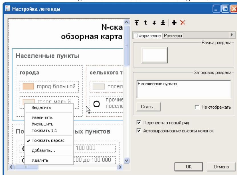
Рисунок 20.6. Редактор легенды
