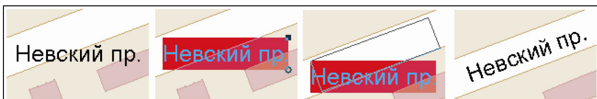
Рисунок 8.17. Поворот текста
