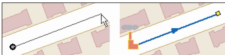
Рисунок 9.6. Нанесение сети
