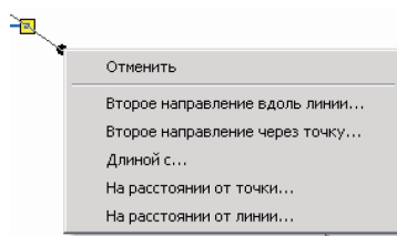
Рисунок 8.9. Контекстное меню
