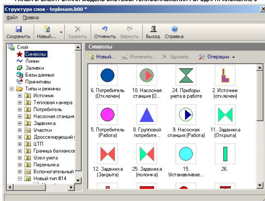
Рисунок 7.7. Библиотека символов
