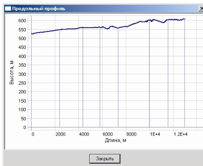
Рисунок 13.10. Продольный профиль
