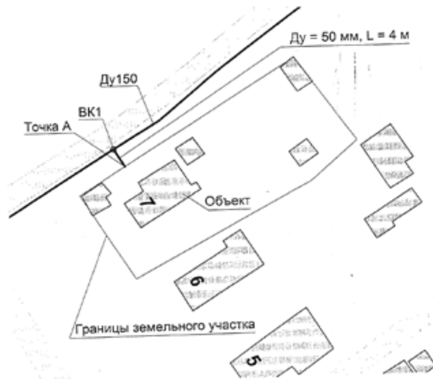
СХЕМА наружной водопроводной сети с указанием точки подключения Объекта
